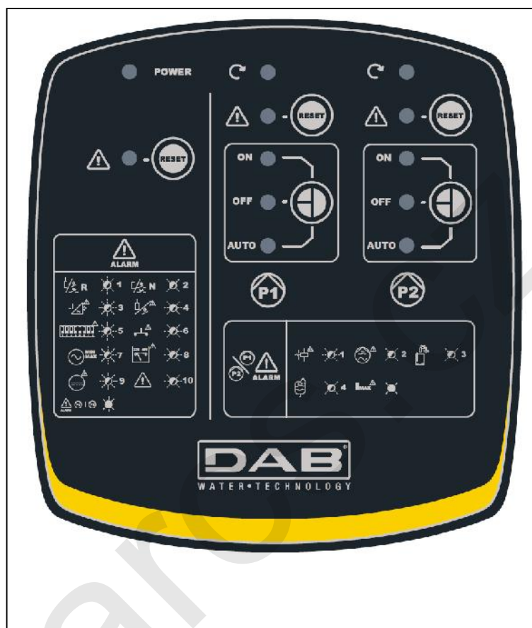
Obrázek 7: P ední část
