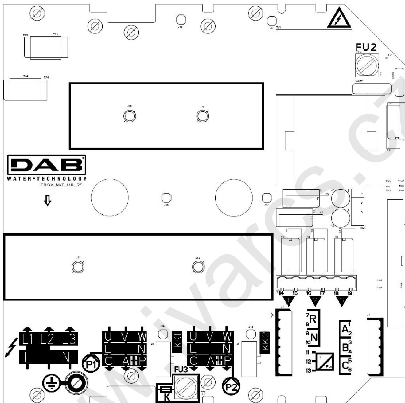
Obrázek 2: P ídavná deska E.BOXU Plus
