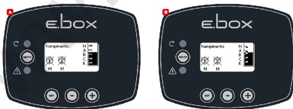
Obrázek 25: Stav systému v režimu pln ní, s plováky nebo hladinovými idly jako řdicími vstupy
