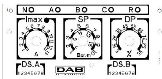
Obrázek 29: Regulování jmenovitého proudu SP a DP
