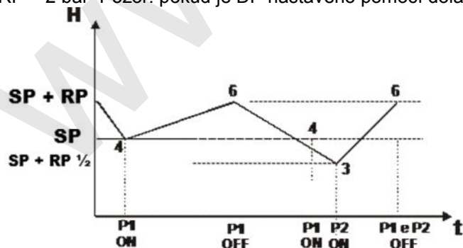
Obrázek 17: Regulace s expanzní nádobou < 100 litr
