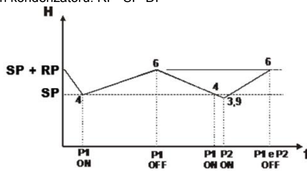
Obrázek 18: Regulace s expanzní nádobou > 100 litr
