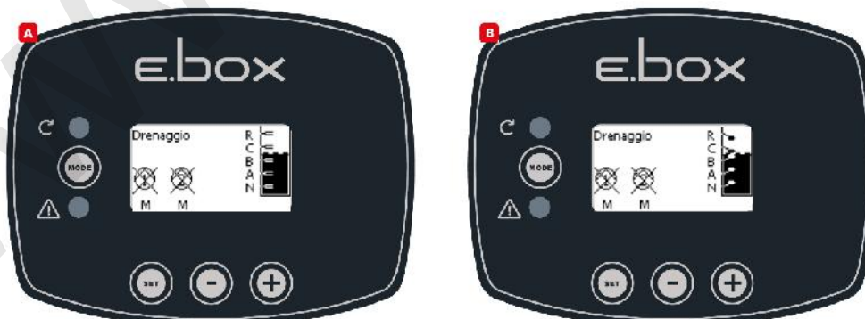
Obrázek 37: Stav systému v režimu vypouštění, A s hladinovými idly. B s plováky
