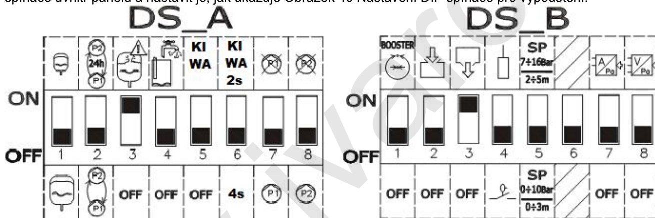
Obrázek 40: Nastavení vypouštění pomocí DIP spínače
