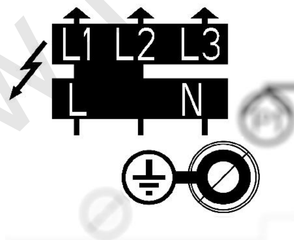
Obrázek 5: Elektrické připojení k napájení
