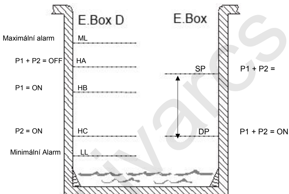
Obrázek 30: Pln ní pomocí hloubkového idla
