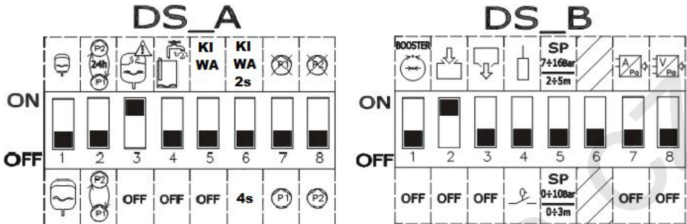
Obrázek 27: Nastavení pomocí DIP spína
