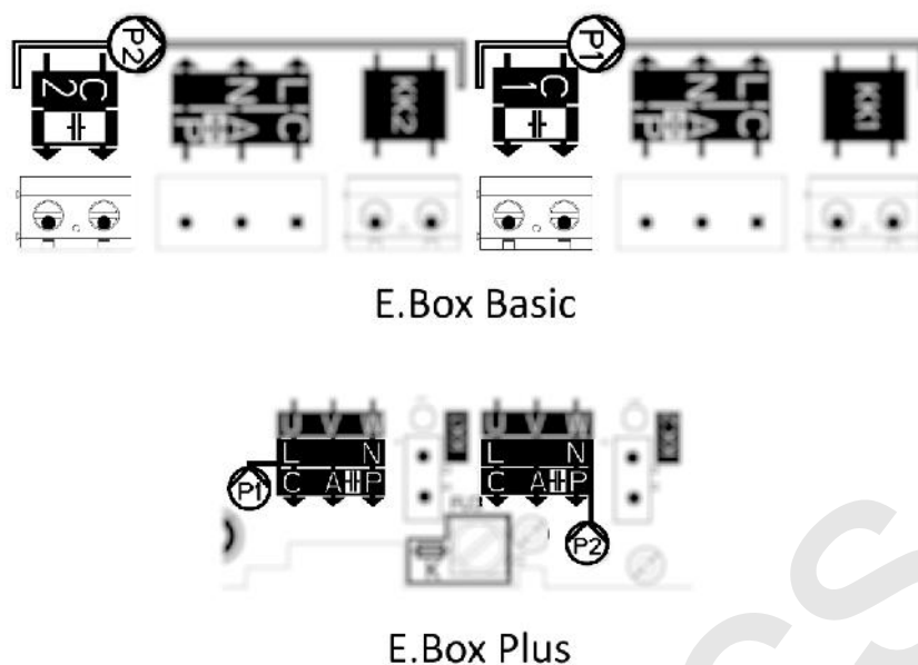
Obrázek 4: P ipojení externích kondenzátorů čerpadla
