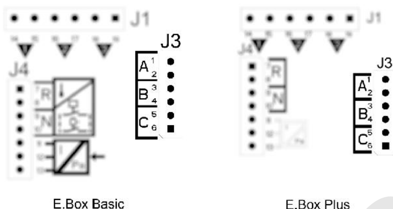
Obrázek 11: Svorky pro p ipojení tlakových spína
