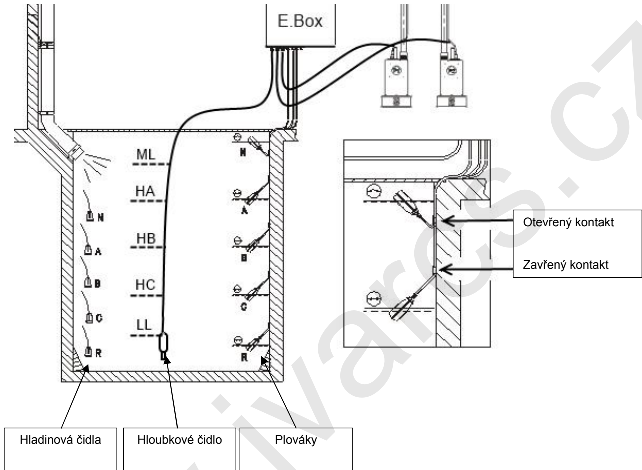
Obrázek 19: Schéma vstup plnění systému
