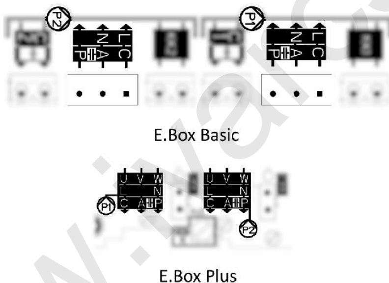
Obrázek 3: Elektrické zapojení čerpadel
